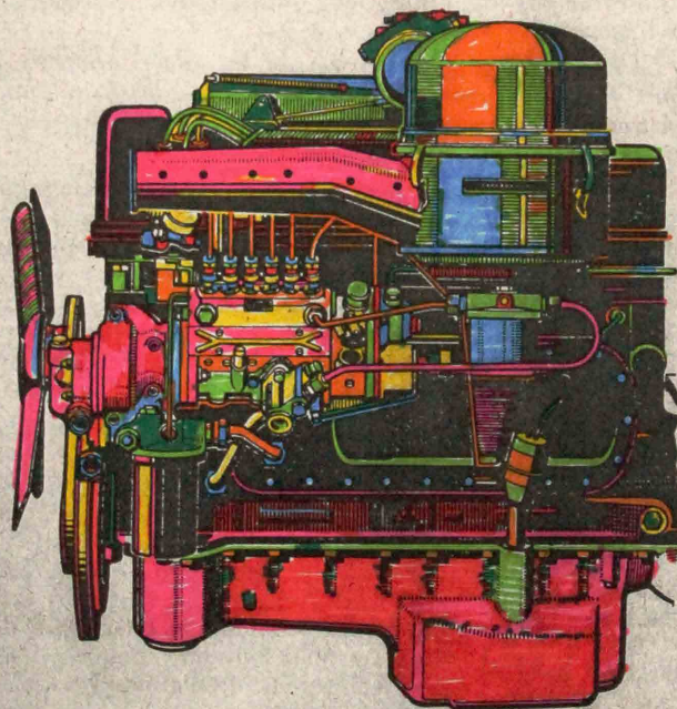
Fig. 298. — Moteur à injection interne d'essence. La pompe d'injection, visible à gauche, s'apparente à celles des moteurs Diesel (Mercedes-Benz)
