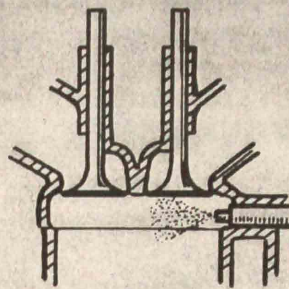
Fig. 297. — Carburation interne : injection dans la chambre de combustion
