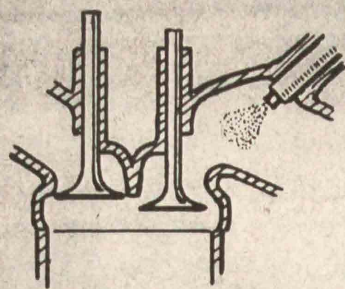
Fig. 296. — Carburation externe : injection dans la tubulure d'admission
